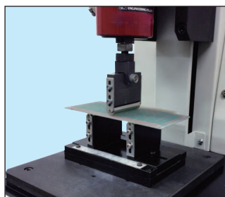
基板曲げ試験
