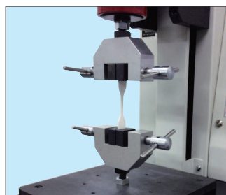
樹脂引張試験
