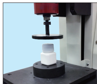
容器圧縮試験
