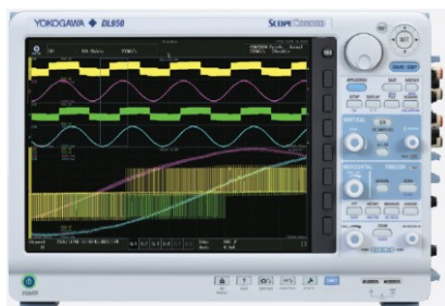
プラグインモジュール (全21種類) 本体に最大8枚のプラグインモジュールを 実装できます。
