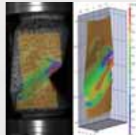
座屈試験
