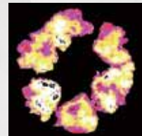
温度解析
