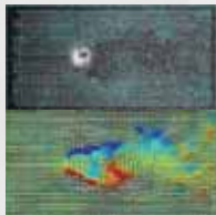
流体解析
