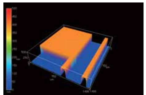
反射分光膜厚測定
