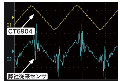
電流を正確に測定する優れたノイズ耐性 PW6001 + CT6904
