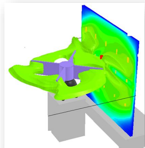
4翼パドルの攪拌解析
