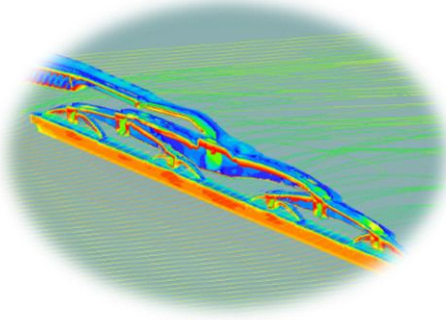
ワイパー空力解析
