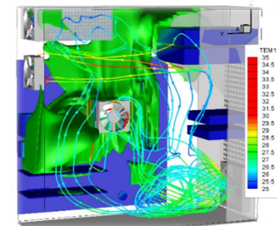
PC筐体内熱流動解析
