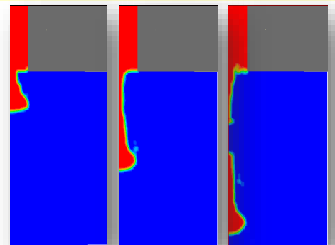
インク液滴吐出解析
