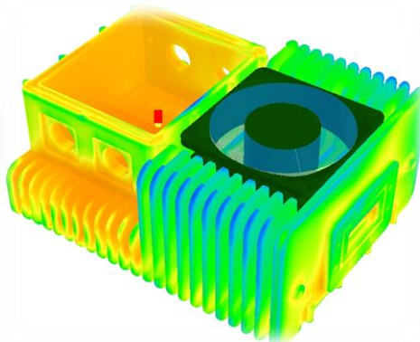
パワーサプライ装置熱解析
