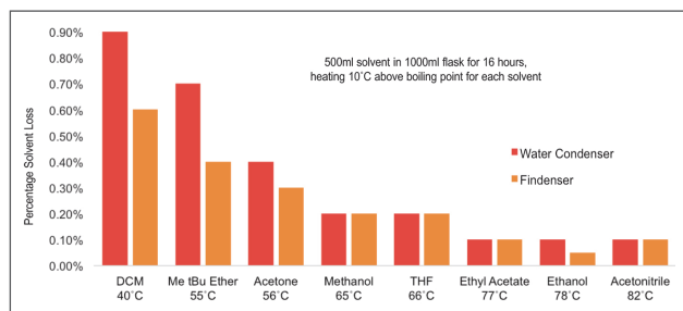
図：一般的な水冷式コンデンサーとの比較
