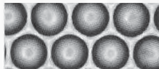
▲マイクロスフェアアレイ微細穴加工 材質：アクリル Φ0.3mm×d0.3mm
