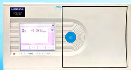
堀場製作所 オゾン濃度測定装置
